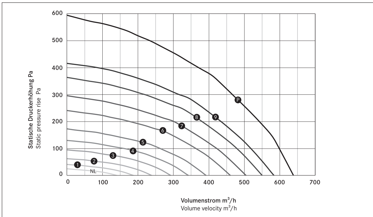
Abb. Luftleistungskennlinien PUXA Fig. Air performance curves PUXA
