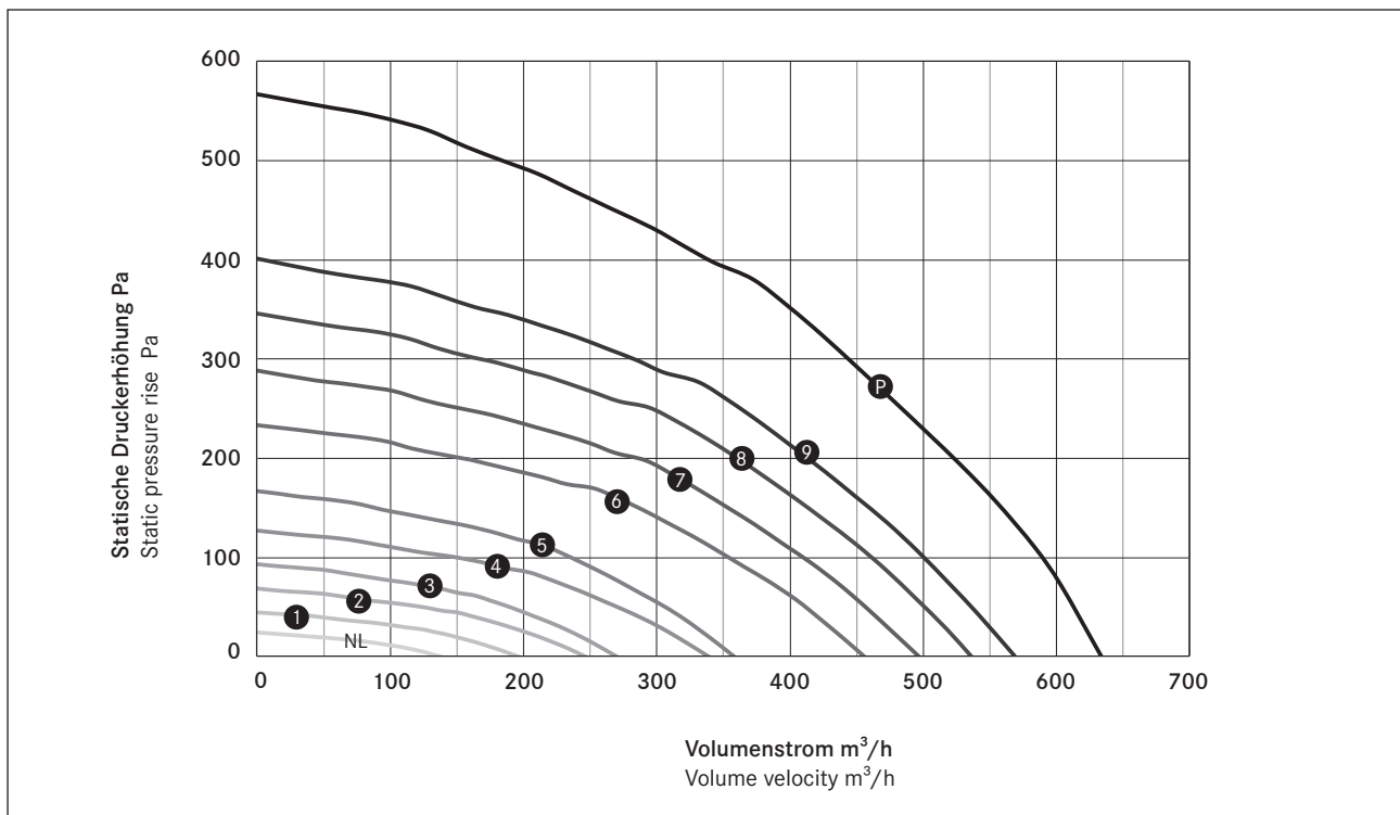
Abb. Luftleistungskennlinien PURSA
